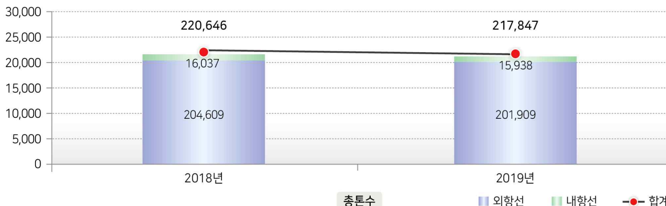
<전년대비 울산항 입항 선박 총톤수 현황>
